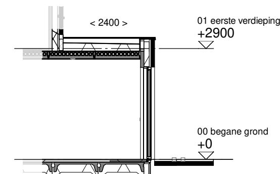
Doorsnede schaal 1:100
