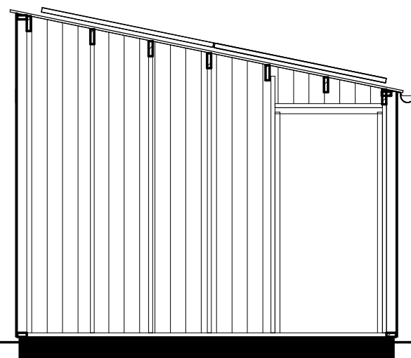
Doorsnede B-B
