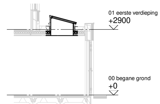
Doorsnede schaal 1:100
