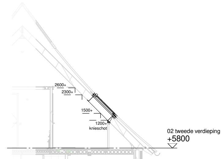
Doorsnede schaal 1:100
