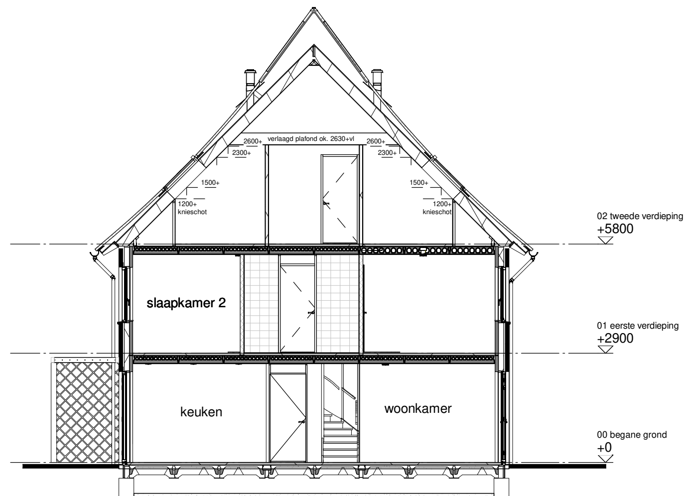
Doorsnede B
