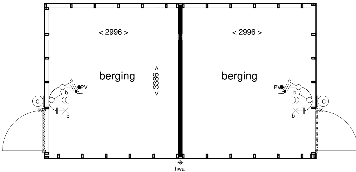
Begane grond
