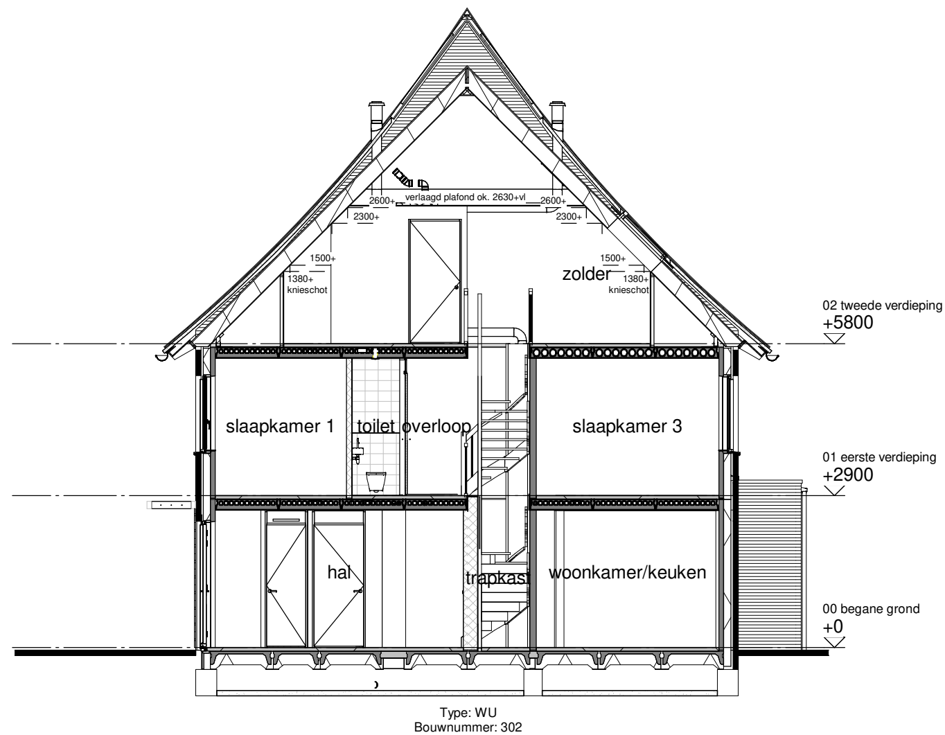
Doorsnede A
