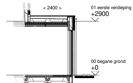
Doorsnede schaal 1:100
