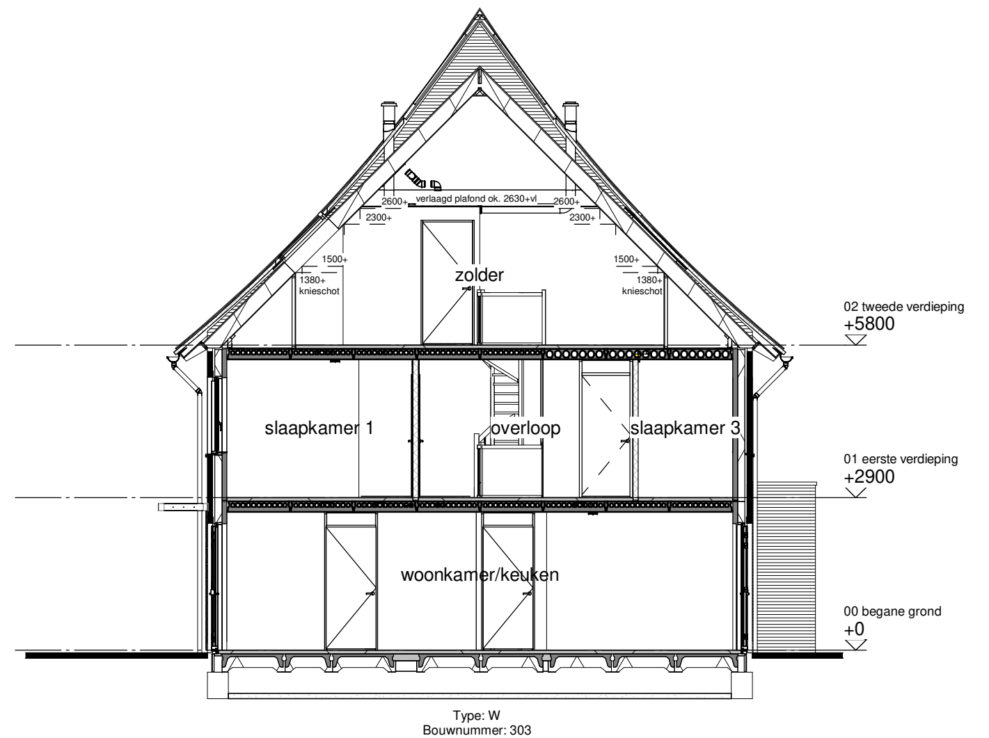
Doorsnede B
