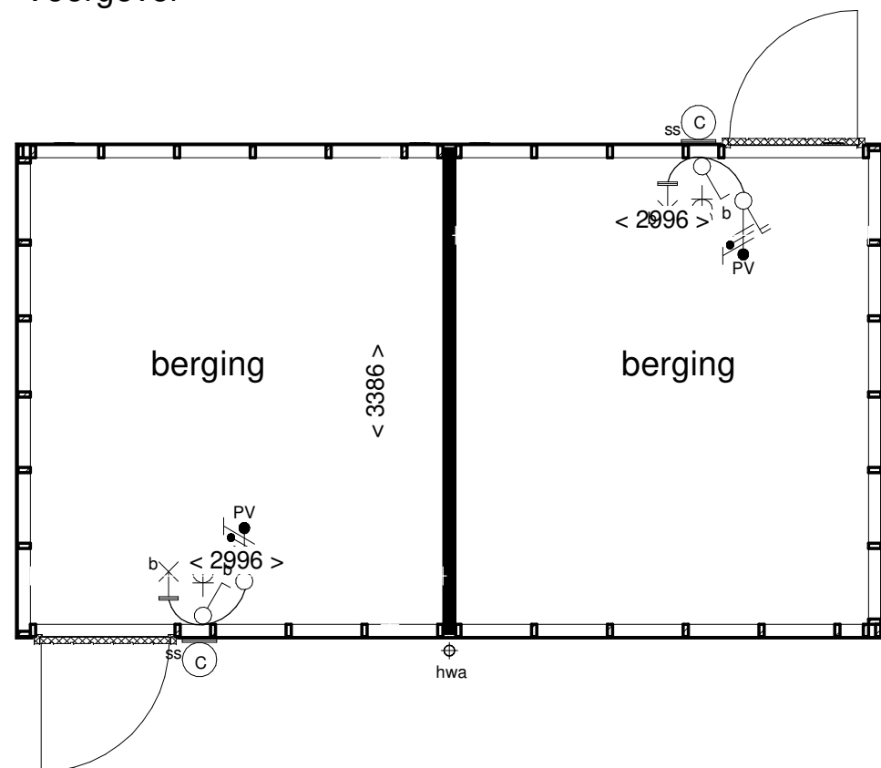
Begane grond
