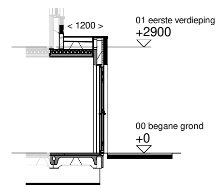
Doorsnede schaal 1:100
