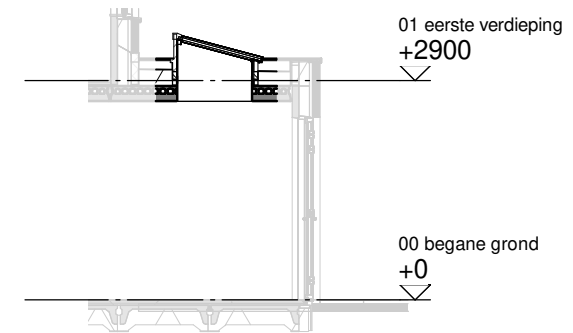
Doorsnede schaal 1:100
