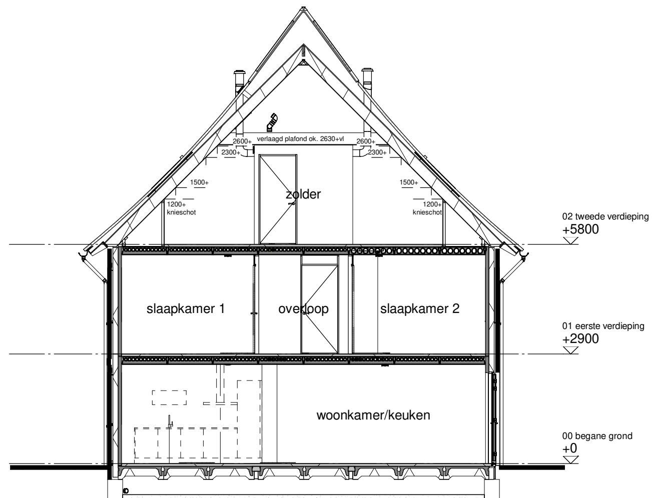
Doorsnede B
