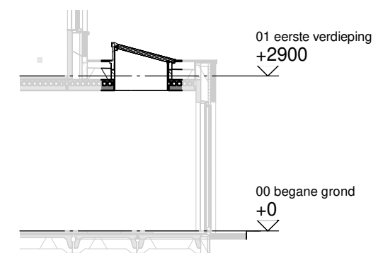
Doorsnede schaal 1:100
