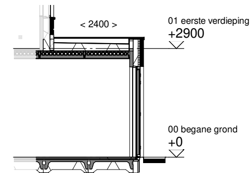
Doorsnede schaal 1:100
