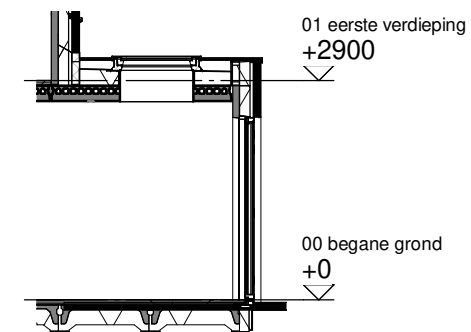
Doorsnede schaal 1:100
