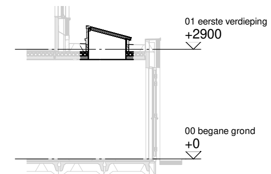
Doorsnede schaal 1:100
