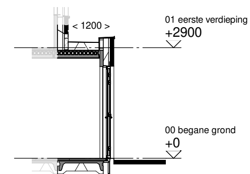
Doorsnede schaal 1:100
