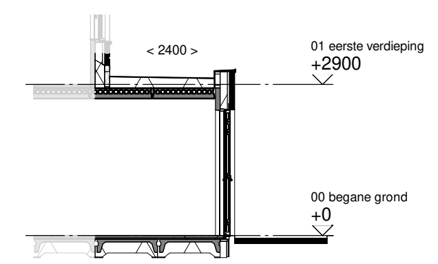
Doorsnede schaal 1:100
