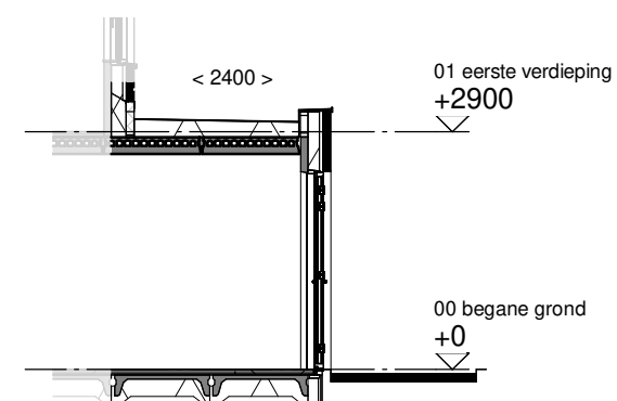
Doorsnede schaal 1:100
