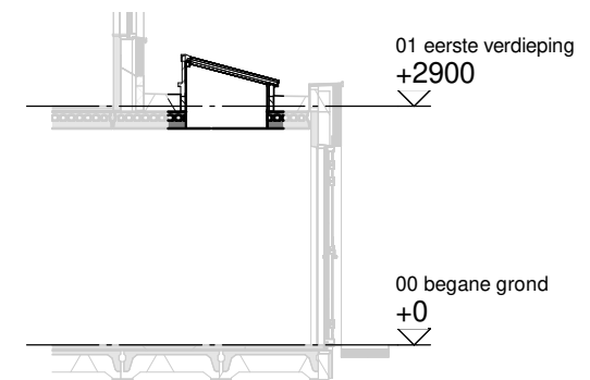
Doorsnede schaal 1:100
