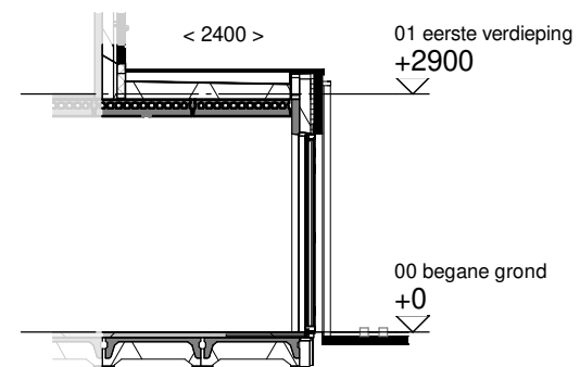
Doorsnede schaal 1:100
