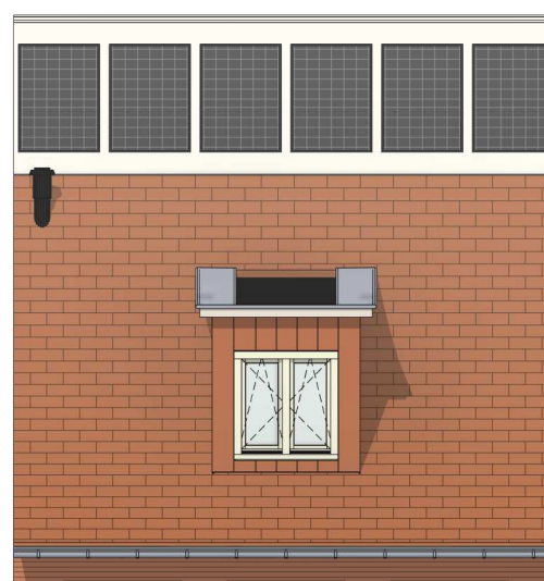
Voorgevel schaal 1:100
