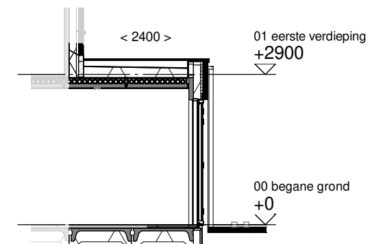
Doorsnede schaal 1:100
