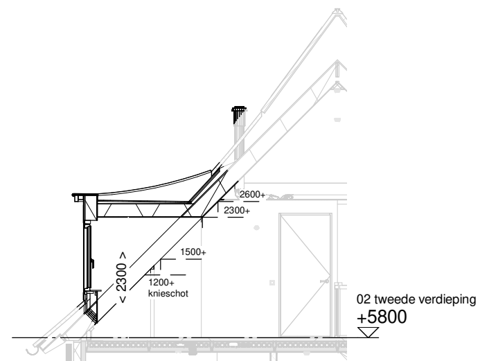
Doorsnede schaal 1:100
