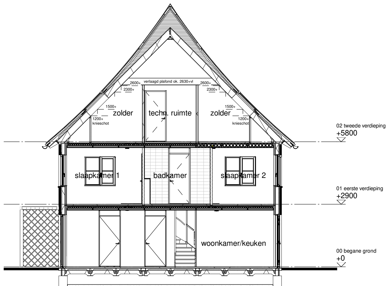
Doorsnede A
