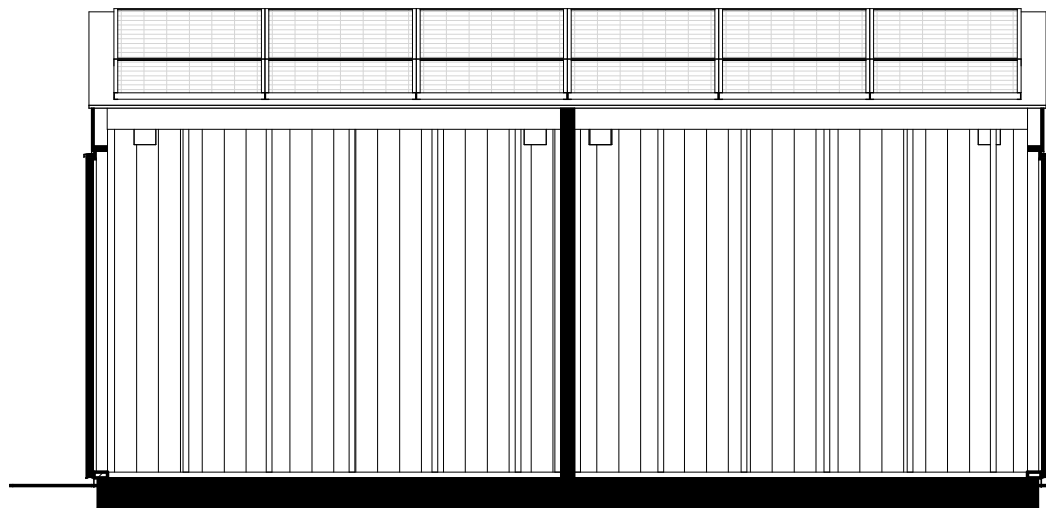
Doorsnede A-A
