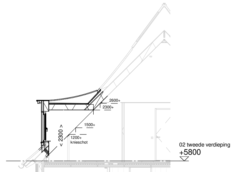
Doorsnede schaal 1:100
