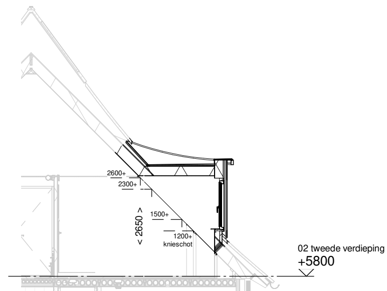
Doorsnede schaal 1:100
