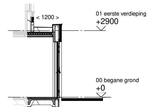
Doorsnede schaal 1:100
