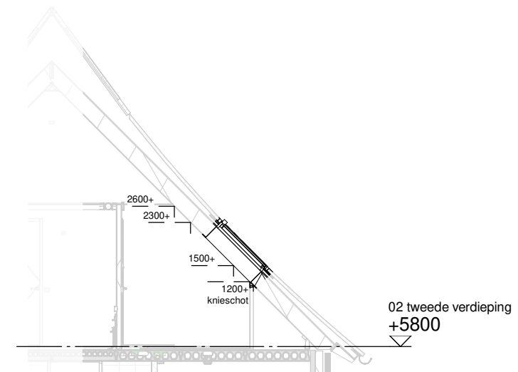
Doorsnede schaal 1:100
