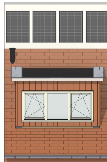
Achtergevel schaal 1:100
