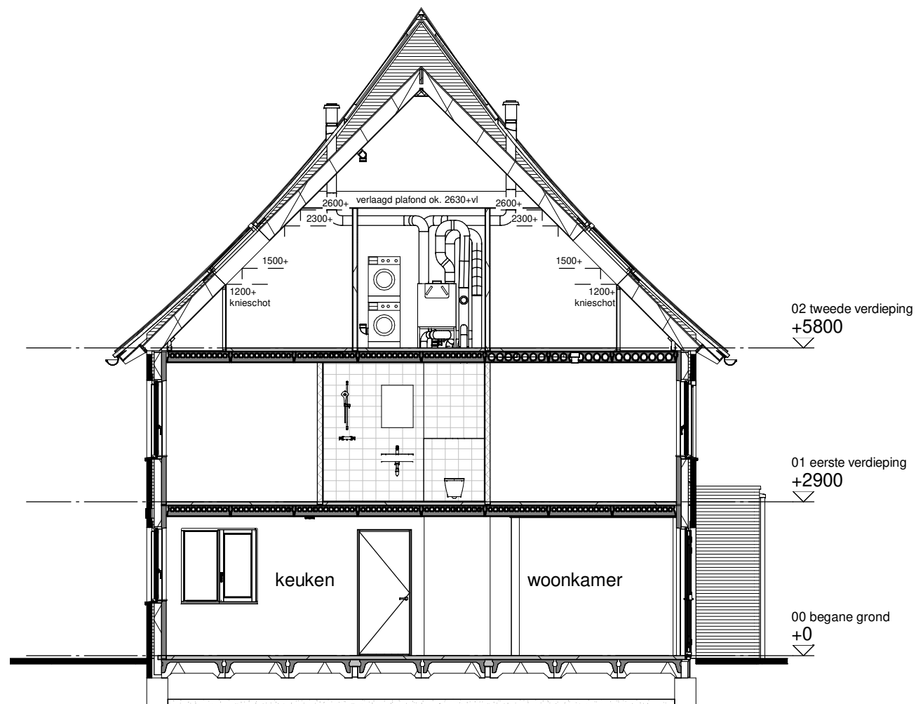
Doorsnede A
