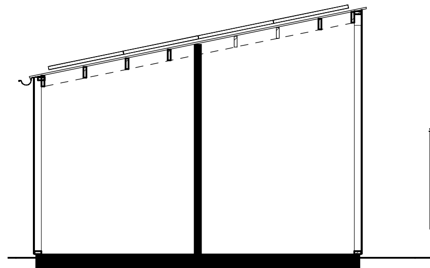
Doorsnede B-B
