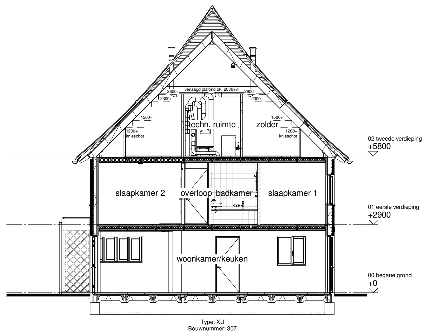
Doorsnede A
